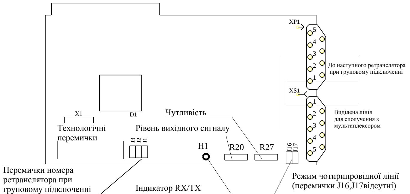
Рисунок 2 – Розташування основних елементів, режим чотирипровідної лінії
