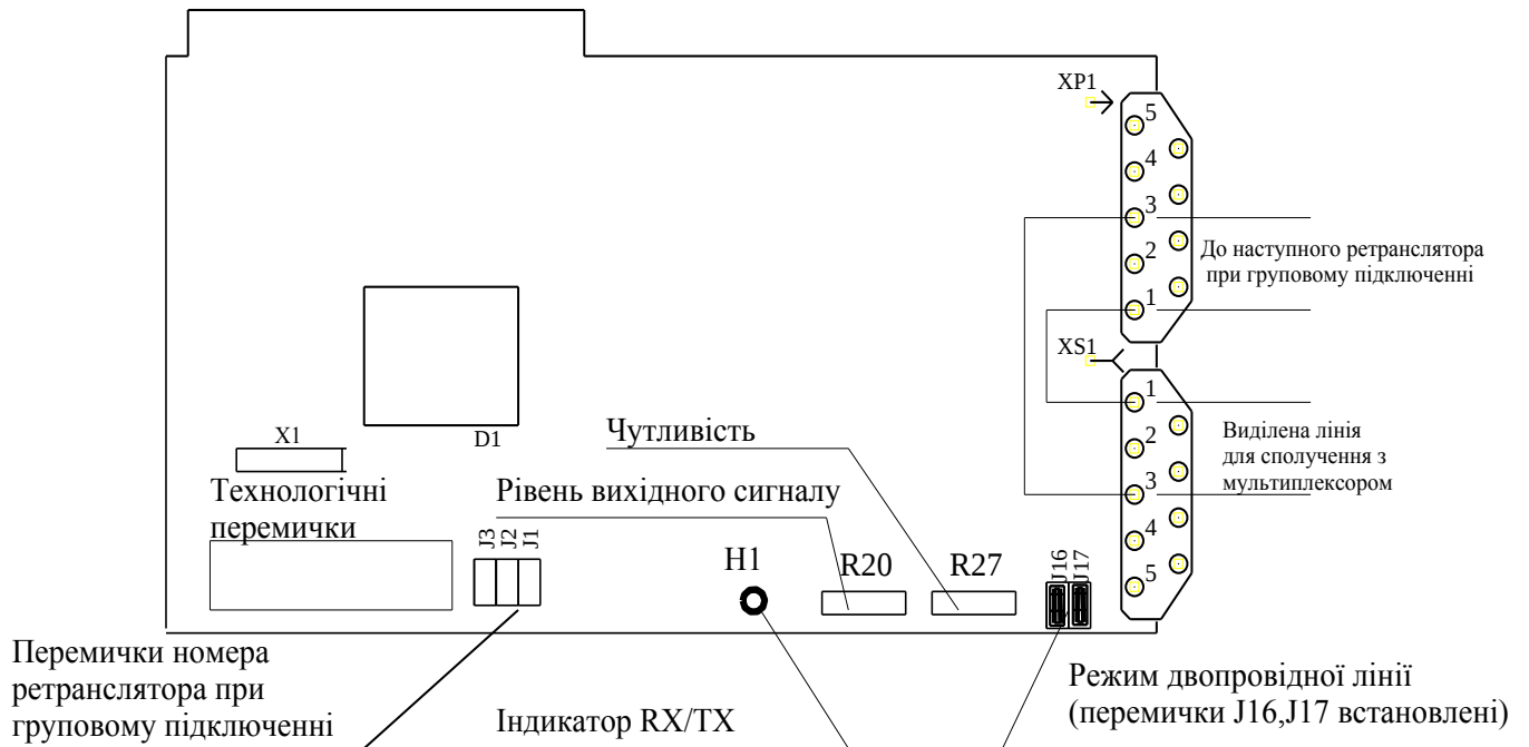
Рисунок 1 – Розташування основних елементів, режим двопровідної лінії
